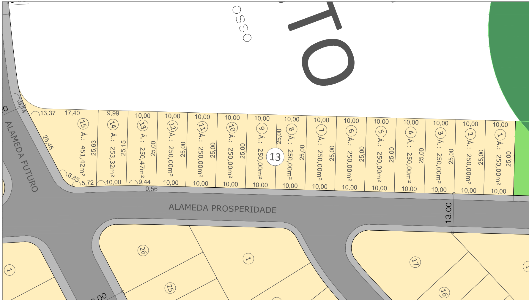
Parcelamento Detalhe: Quadra 13 Sem Escala
