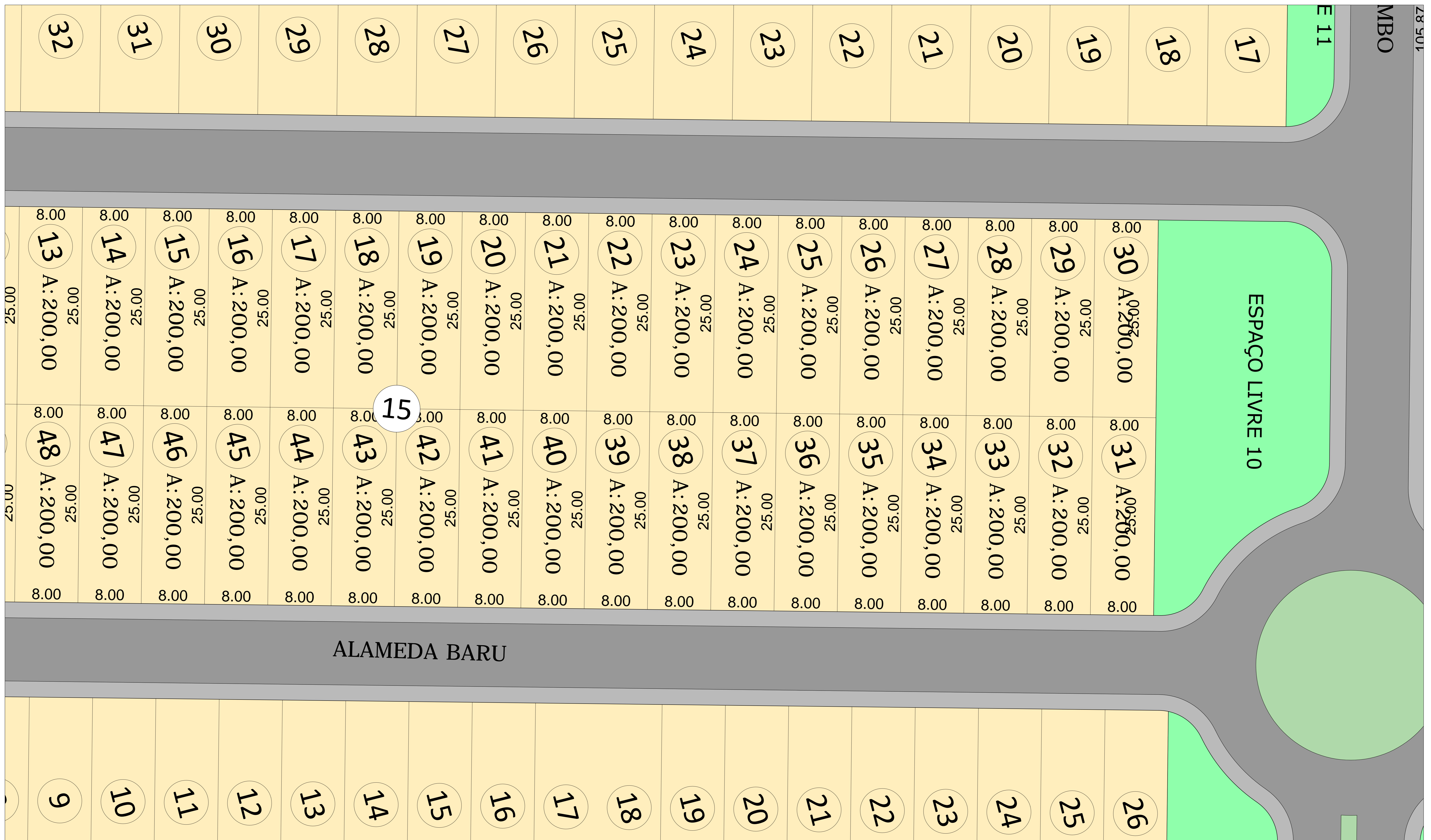
Detalhe: Quadra 15 - Lotes do 13 ao 30 e do 31 ao 48 Sem Escala
